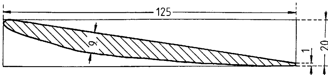
SCHNITT 3
