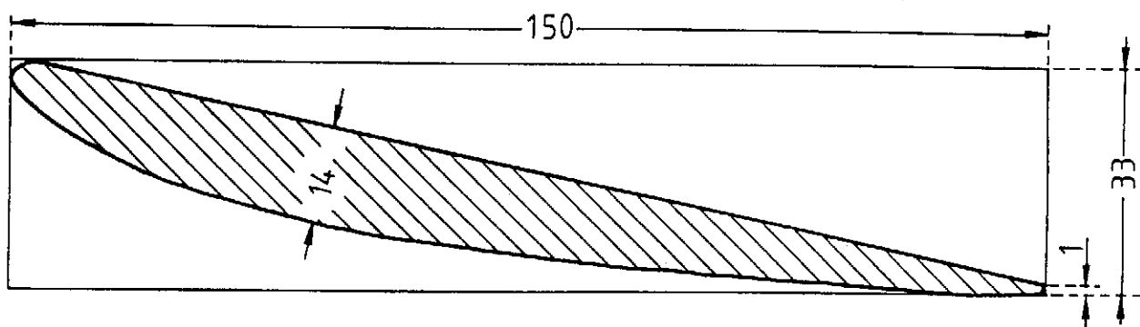
SCHNITT 5
