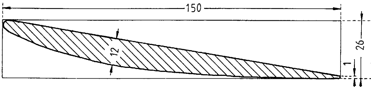
SCHNITT 3
