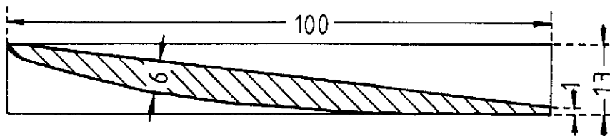
SCHNITT 2
